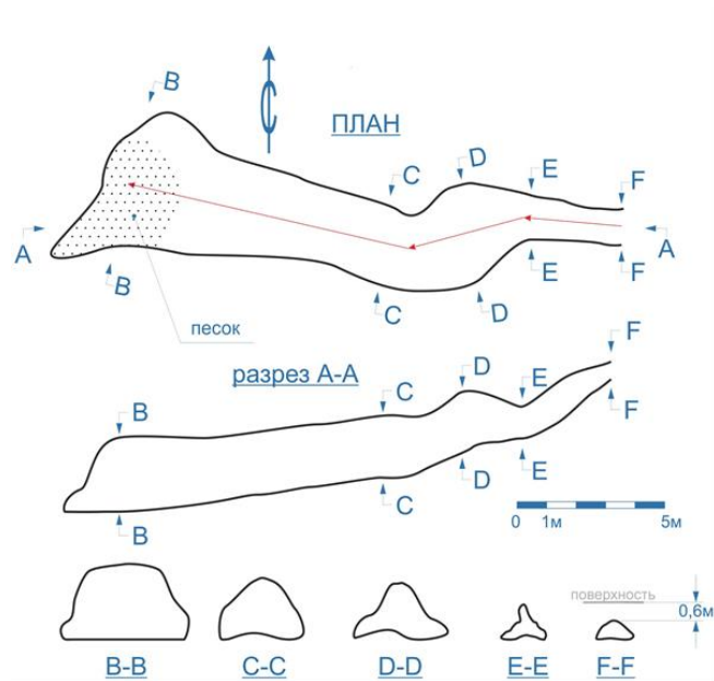
Рис. 3. План та розрізи карстової порожнини в середині колишнього Татарбунарського замку
